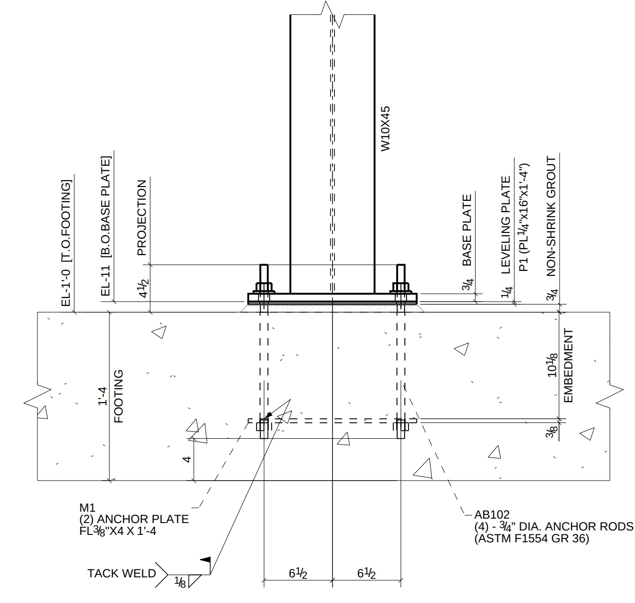
4 BASE DETAIL - 4 SCALE: 1:9
