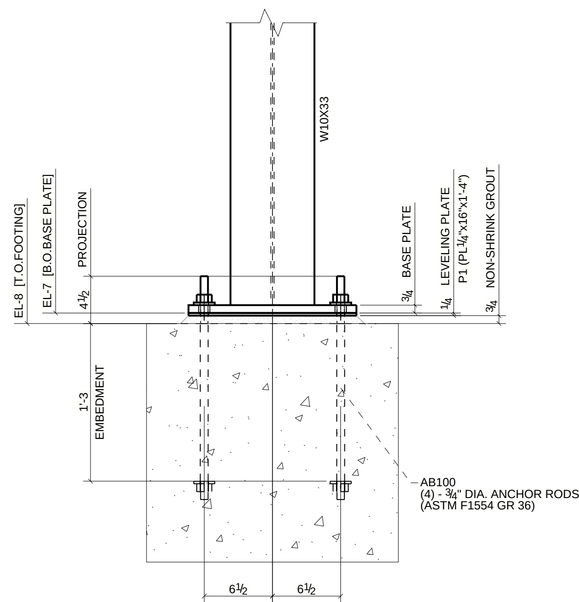
1 BASE DETAIL - 1 SCALE: 1:9
