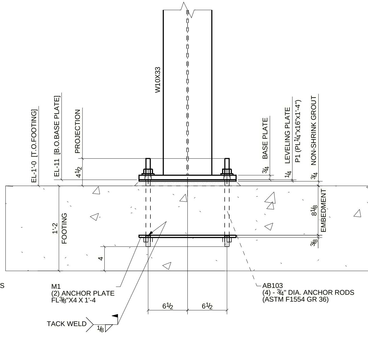
2 BASE DETAIL - 2 SCALE: 1:9
