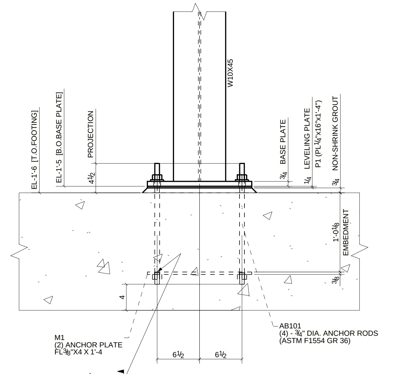
5 BASE DETAIL - 5 SCALE: 1:9
