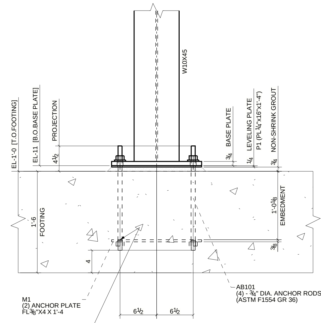
3 BASE DETAIL - 3 SCALE: 1:9
