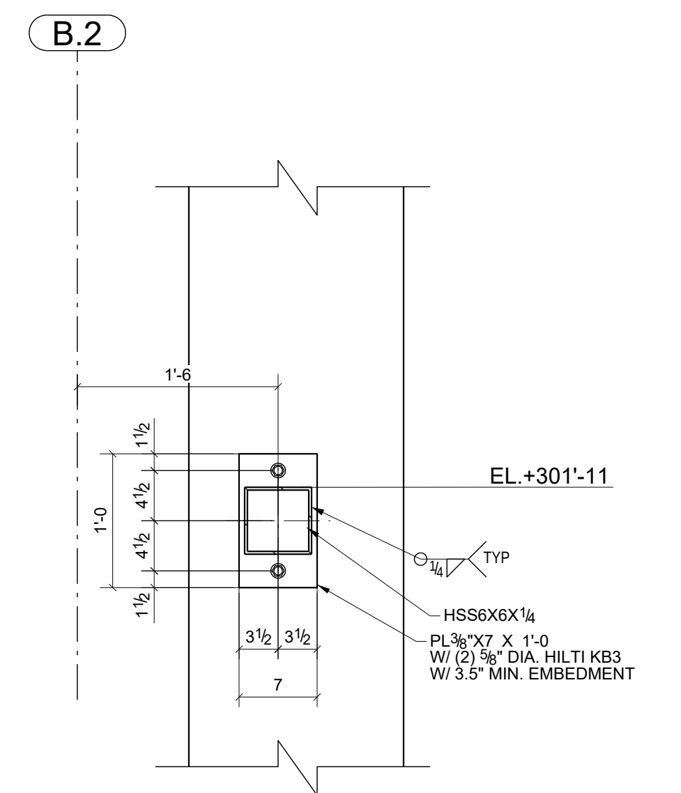
3 SECTION DETAIL SCALE: 1:12
