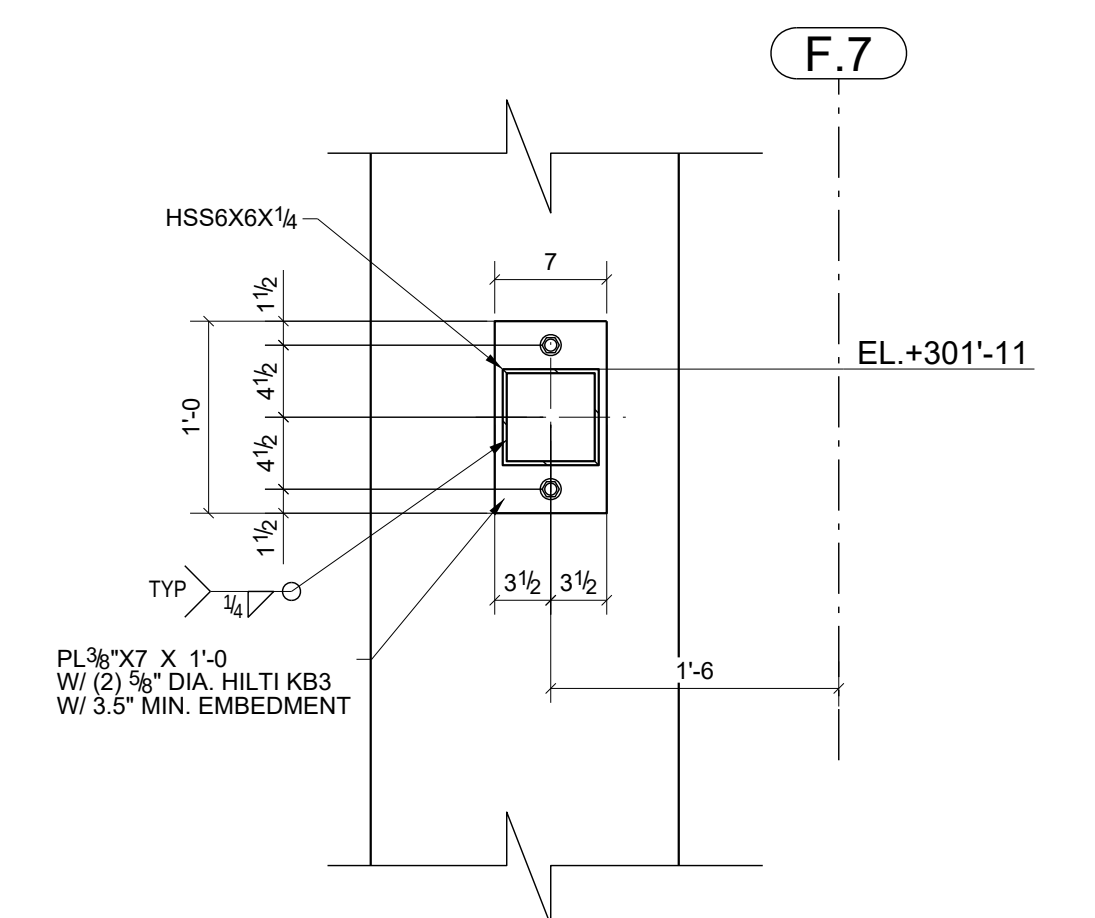
3 SECTION DETAIL SCALE: 1:12
