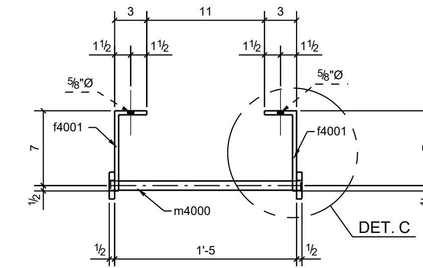
B - B
