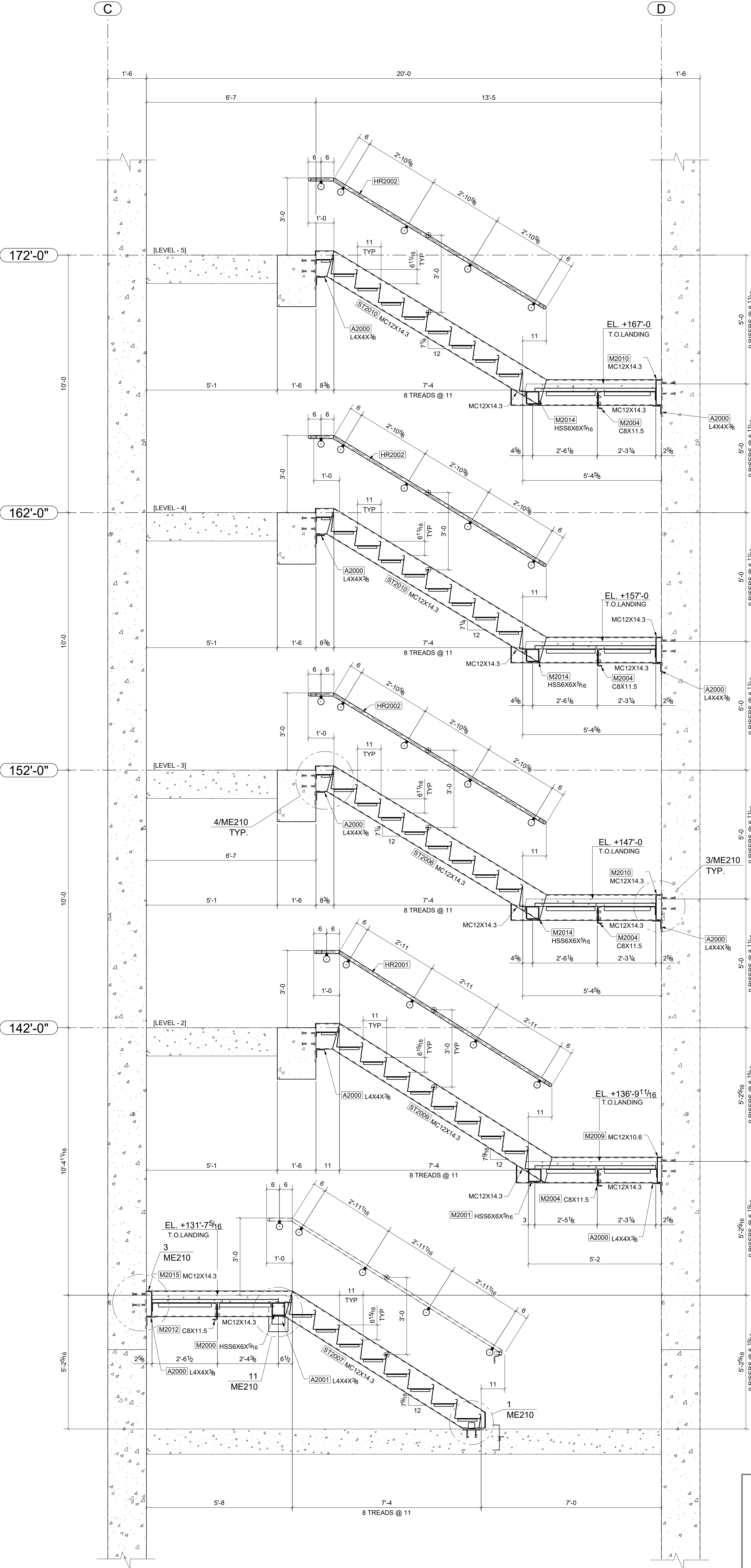
1 SECTIONAL ELEVATION - STAIR #B SCALE: 1:24
