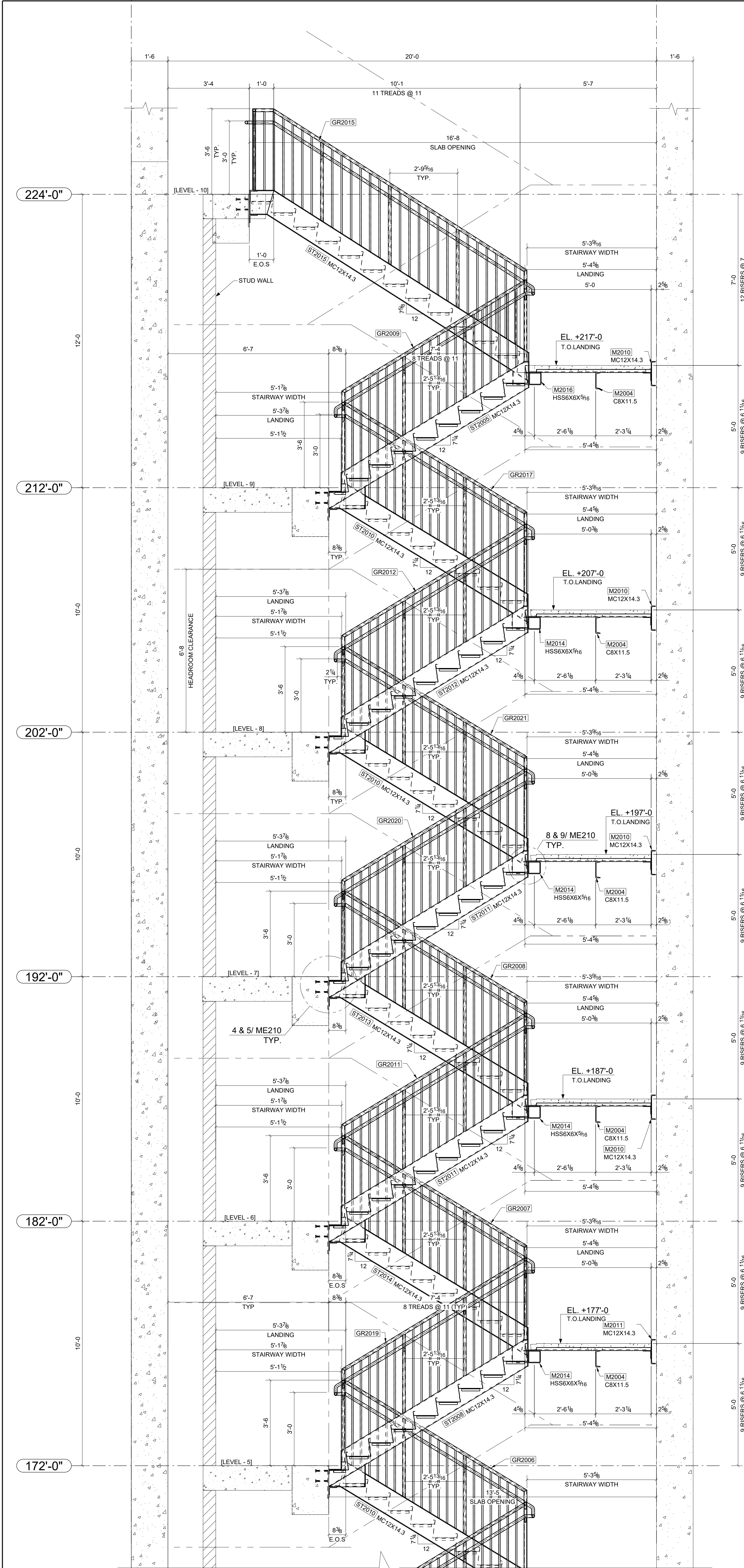
1 SECTIONAL ELEVATION - STAIR #B SCALE: 1:24
