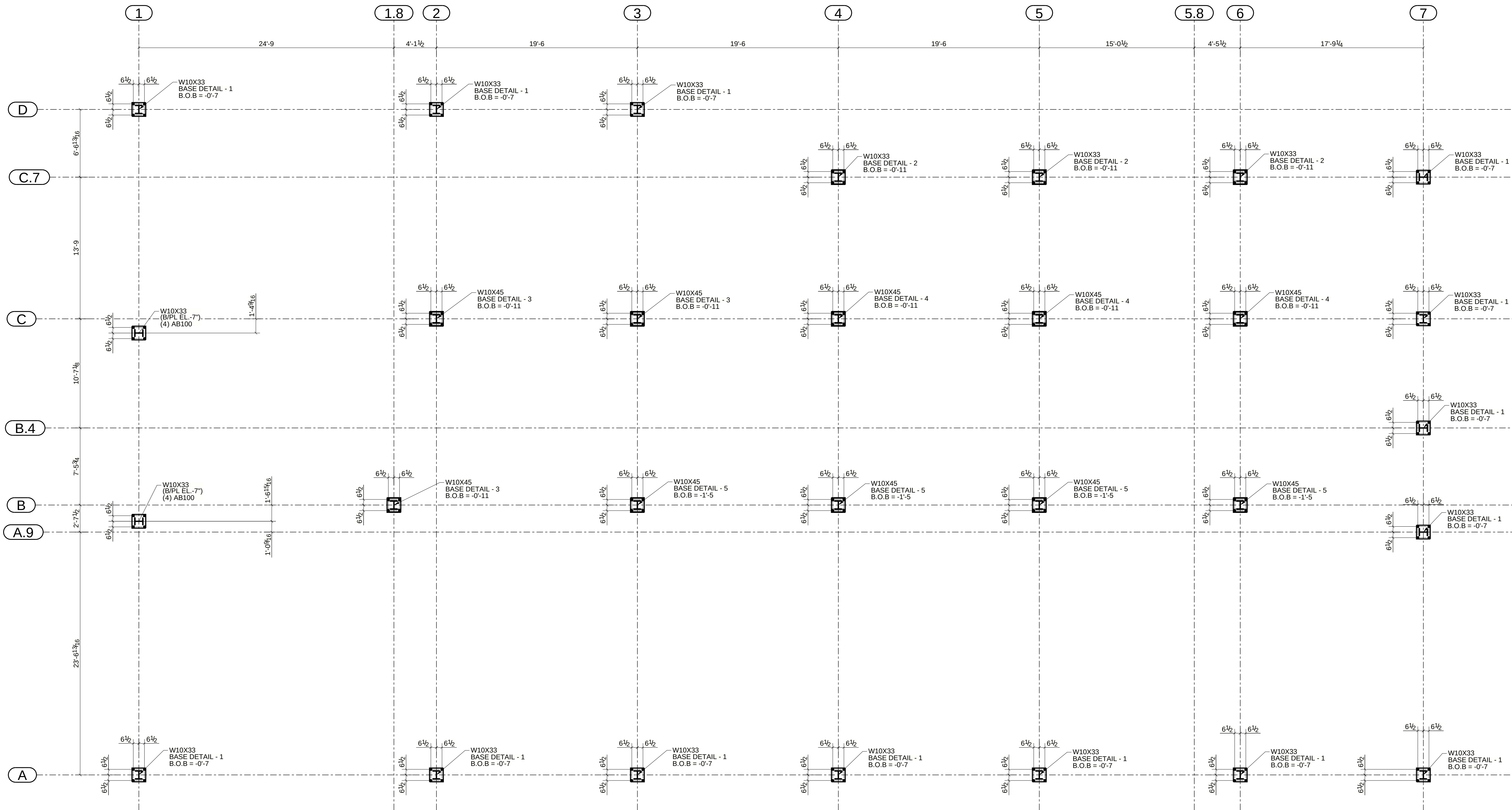
1 ANCHOR ROD LAYOUT PLAN SCALE: 1:64
